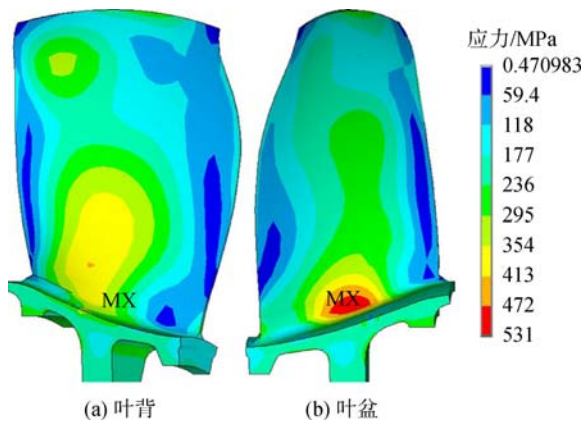
图 8 不考虑轮盘的优化后应力分布验证
