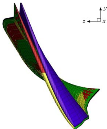
图3 热态叶型到冷态叶型求解结果
