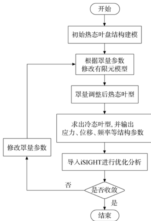
图5 罩量调节优化流程图
