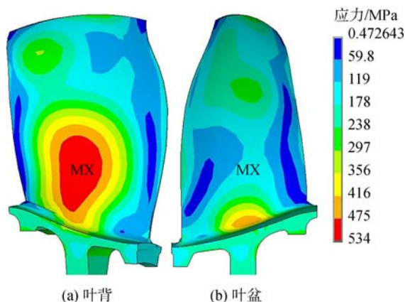
图 6 优化前应力分布
