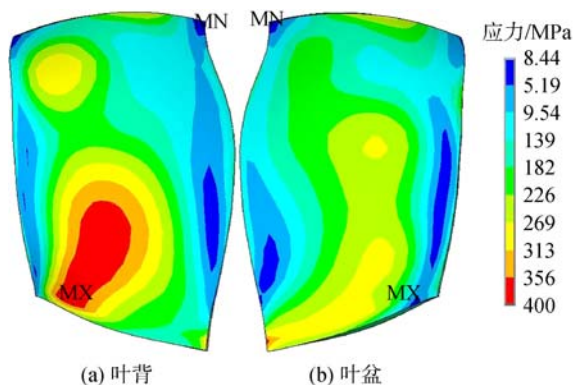
图 7 不考虑轮盘的优化后应力分布
