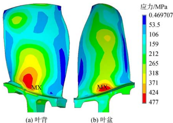
图9 考虑轮盘的优化后应力分布
